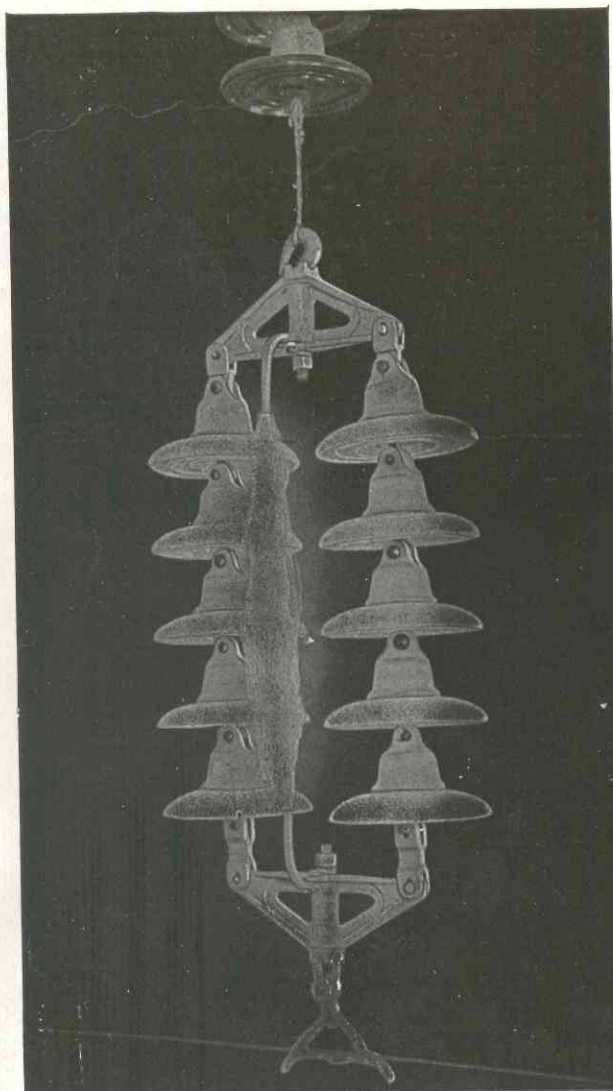
Descarga de un aislador de doble suspensión a 220.000 voltios
