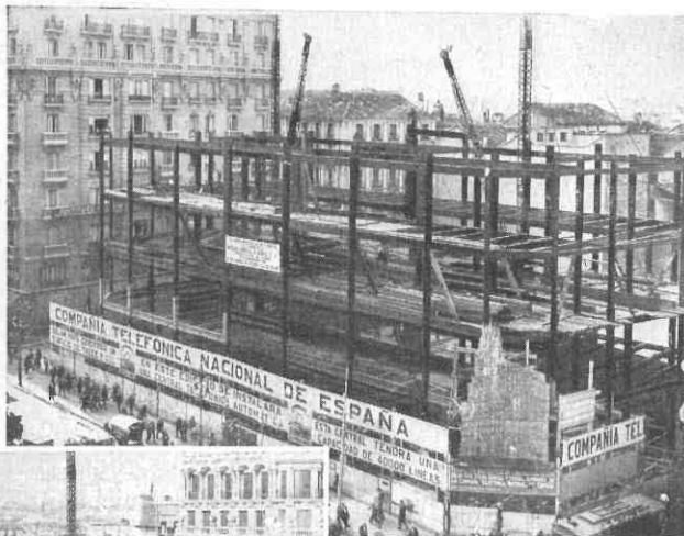
Madrid: Estado de la estructura metálica del edificio que se construye en la Avenida de Pi y Margall, a mediados de junio pasado
