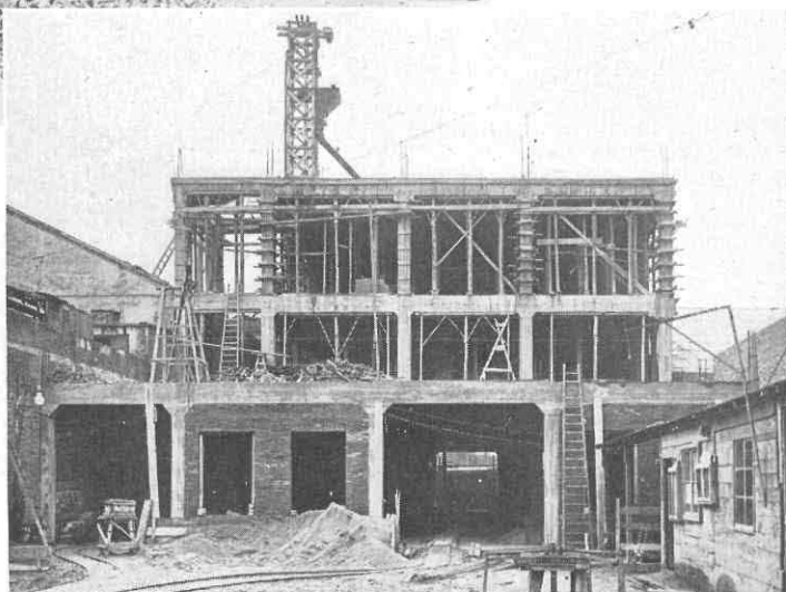
Barcelona: Obras de la fachada posterior de la futura central automática de Arenas
