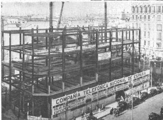
Madrid: Otra perspectiva de la misma obra tomada desde el lado opuesto. Obsérvense las potentes grúas
