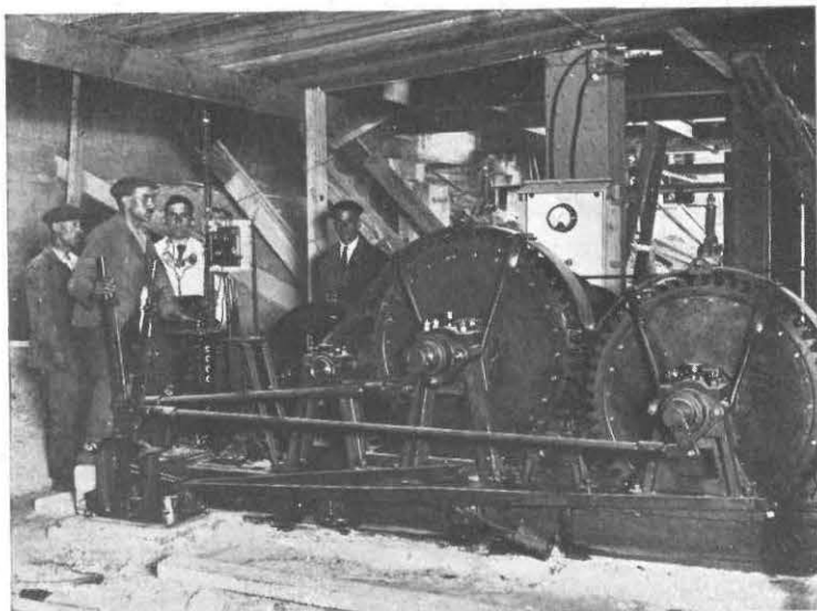
Vista del motor que hace funcionar las grúas instaladas para la elevación y colocación de las vigas y columnas metálicas en las obras del nuevo edificio de la Compañía en Gran Vía
