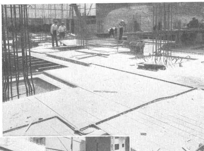
Barcelona: Preparación de la primera planta de la futura central automática de Travesera
