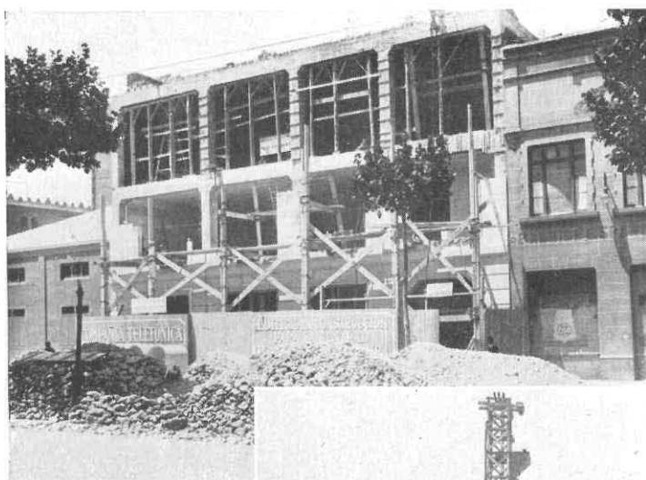
Barcelona: La fachada en construcción de la futura central automática de Arenas
