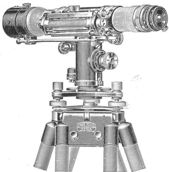
NIVEL ZEISS
