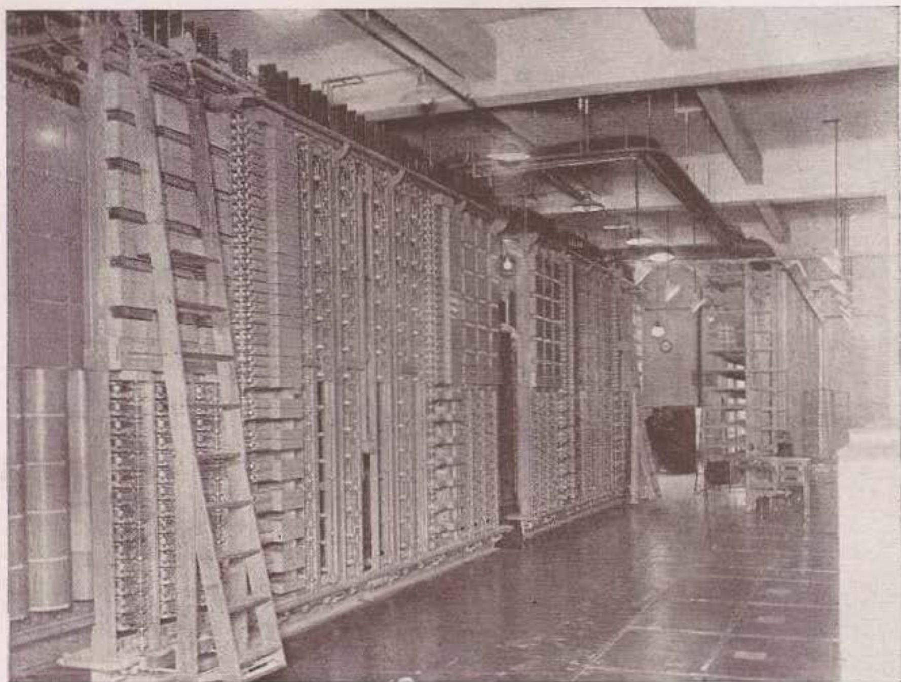
Bilbao. — Equipo automático
