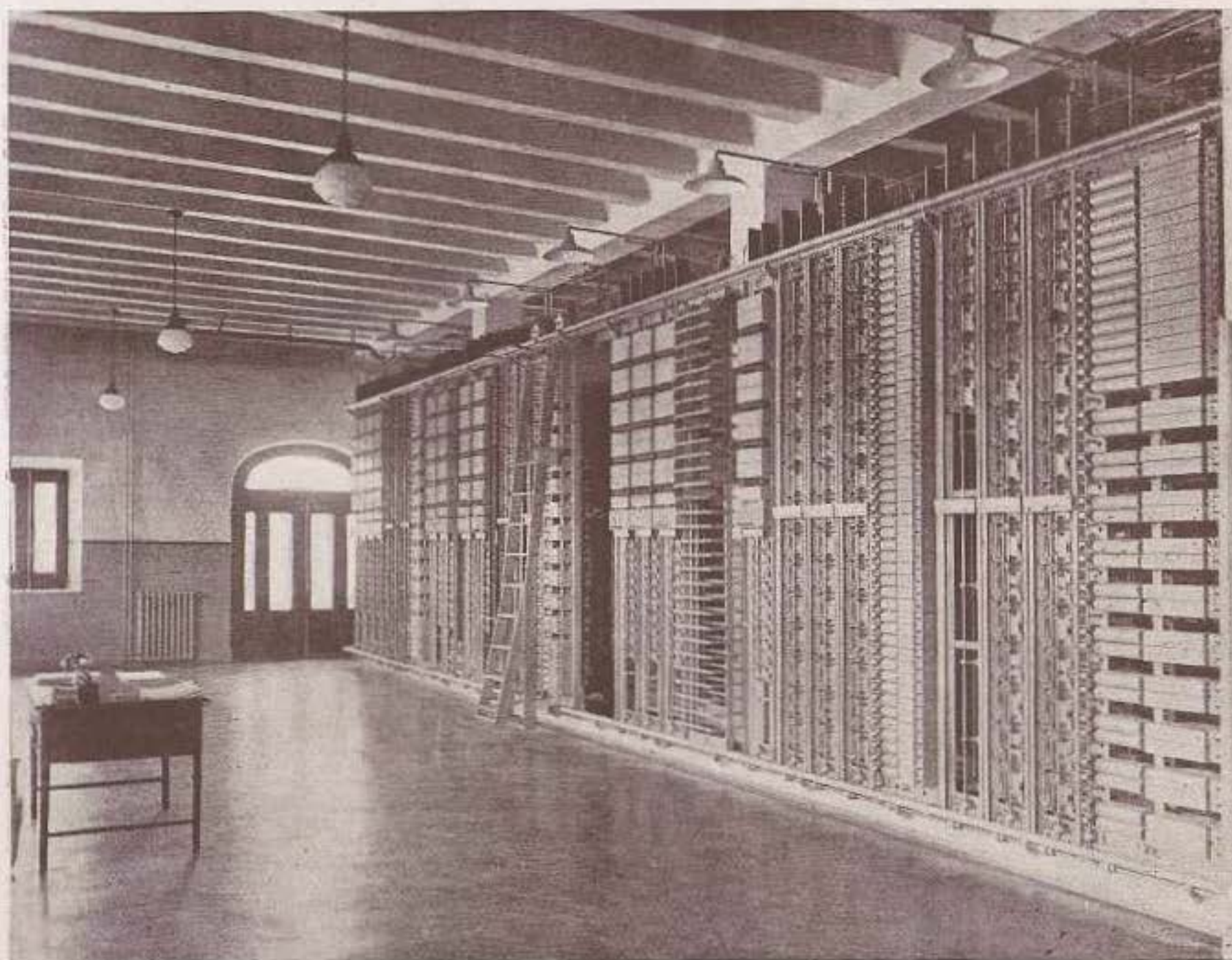
Sevilla. — Vista del equipo automático con los bastidores sin llenar por completo
